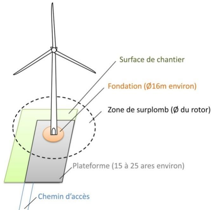
Illustration des emprises au sol d'une éolienne
