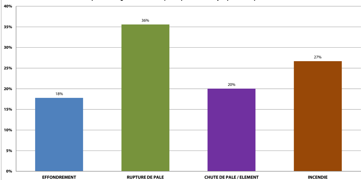
Répartition des événements accidentels sur le parc d'aérogénérateurs français depuis l'an 2000 jusqu'au 30 septembre 2016
